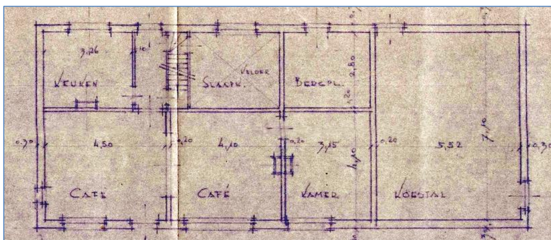
Figuur 8 : Blaudruk van grondplan van café De Jachthoorn en woning. De voorkant langs de Gouden Leeuwstraat is onderaan de tekening (archief Stad Sint-Niklaas)
